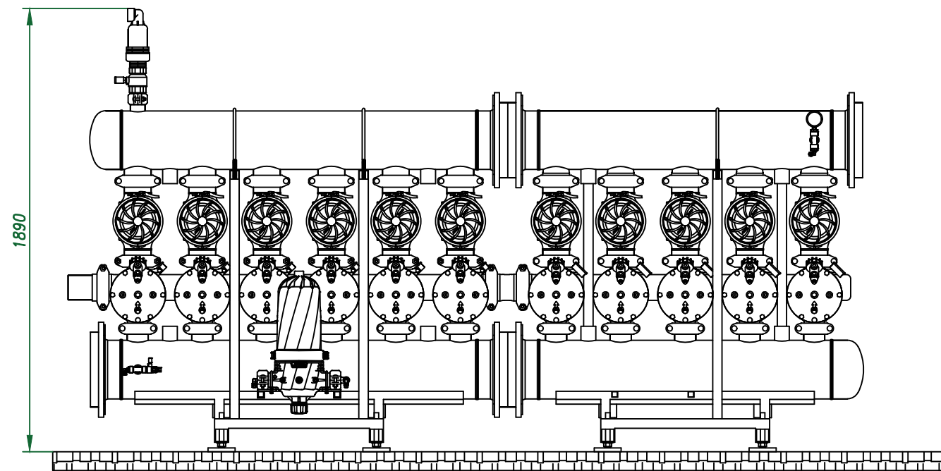
Вид спереди
